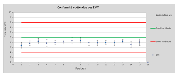
Рис. 13. Аттестация хранилищ для вакцин от +2°C и +8°C ©Cemafrroid
